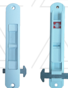
FECHO CONCHA COM GATILHO SEM MOLA
